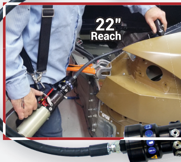
Blind Rivet Adapter DF-SPR/BRAD
